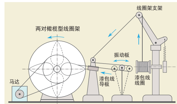
偏转线圈（上）与偏转线圈绕线机的原理图（下）
