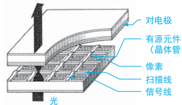
〈有源矩阵驱动方式 (TFT) 的构造〉
