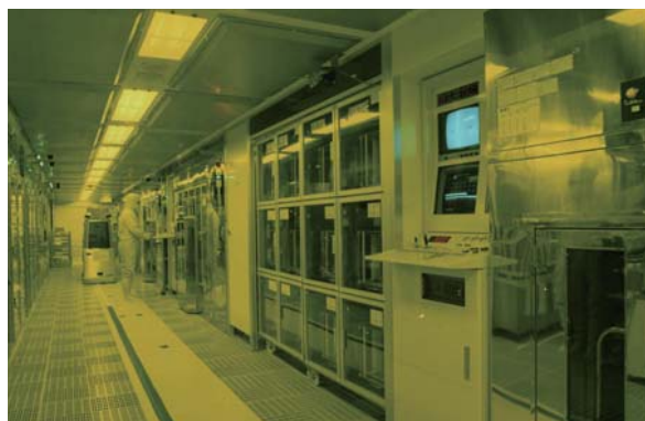
TFT彩色液晶的深加工生产线（天理工厂）
