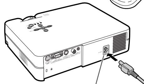
Netzanschluss
