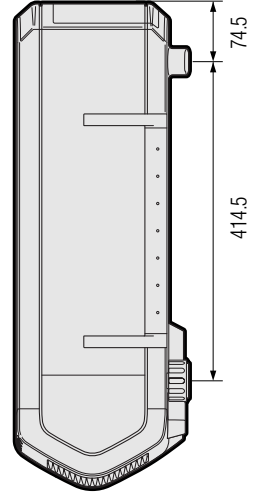
側面
