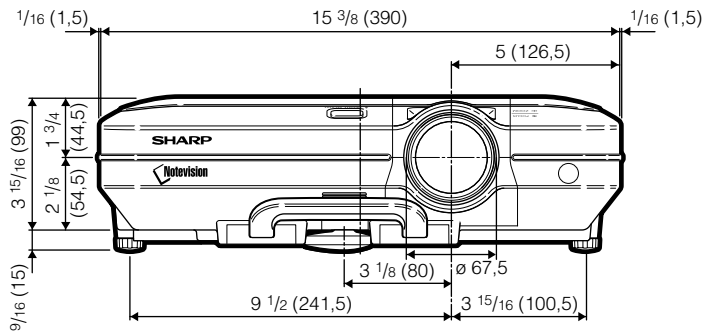
Vooraanzicht
