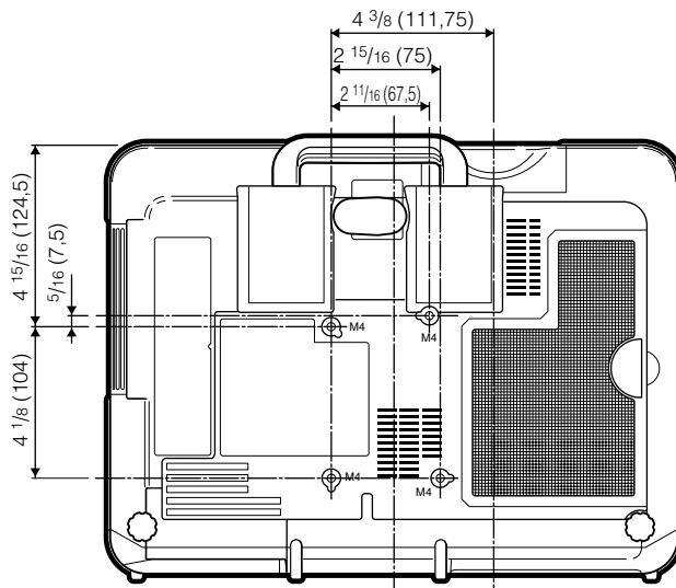
Vista inferiore
