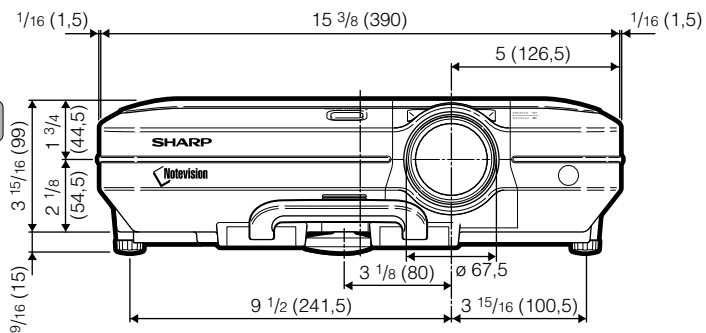
Vista frontale
