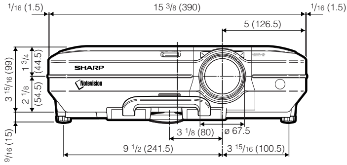
前视图
