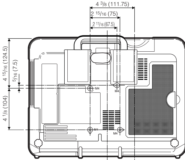
底视图
