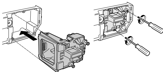
ユーザーサービスネジ
