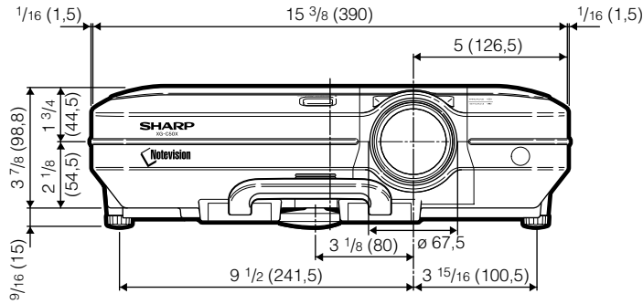
Framifrån
