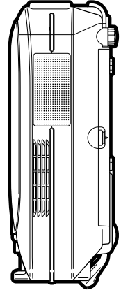
Sidovy
