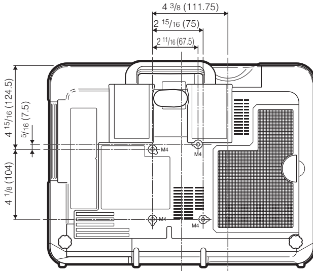
底視圖
