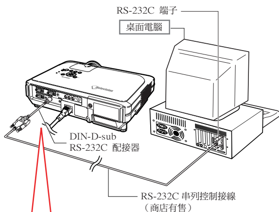
DIN-D-sub RS-232C 配接器
