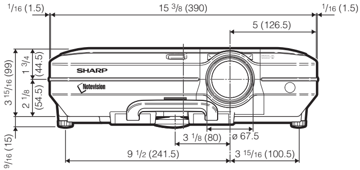
前視圖
