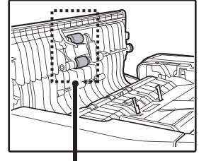
Paperinsyöttötela
