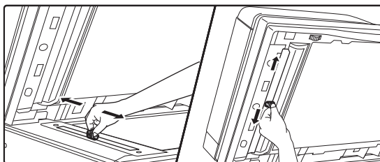
Papíradagoló görgő
