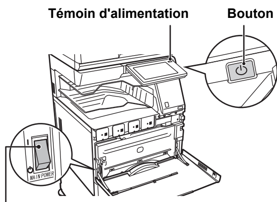
Interrupteur principal
