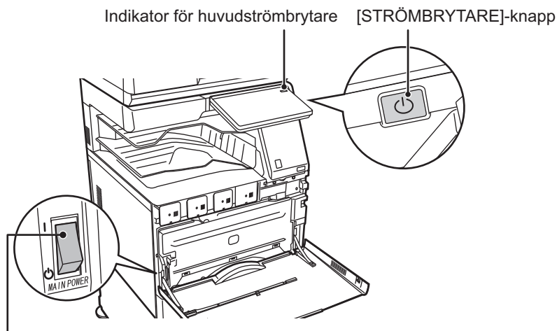
Huvudströmbrytare
