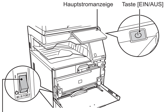
Hauptstromschalter
