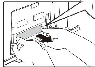
Rolă de alimentare a tăvii manuale
