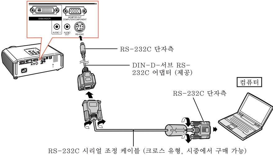
RS-232C 시리얼 조정 케이블 (크로스 유형, 시중에서 구매 가능)
