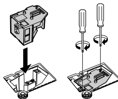
Bevestigingsschroeven
