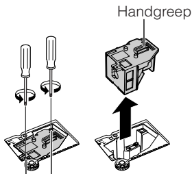
Bevestigingsschroeven
