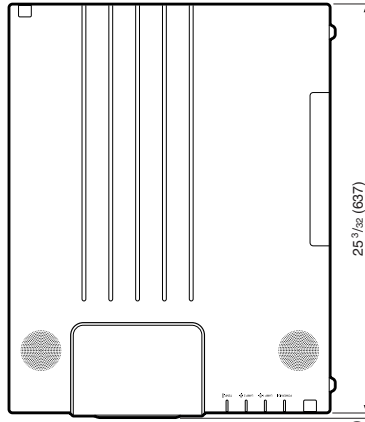
Vista Superior
