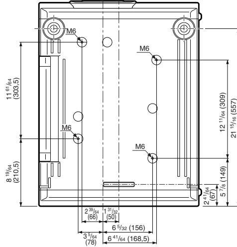
Vista Inferior
